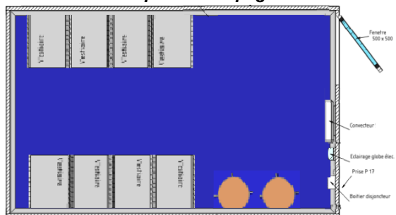
BDV8 - Vestiaire pour 8 compagnons
