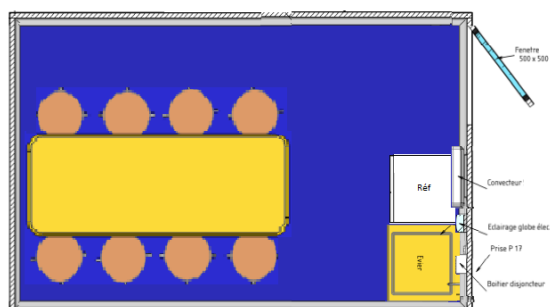
BDR8 - Réfectoire pour 8 compagnons
